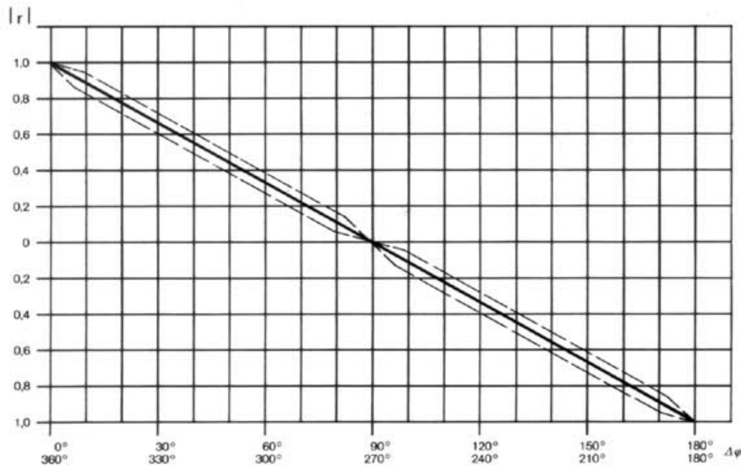
Korrelationsgrad r als Funktion des Differenzphasenwinkels \Delta\varphi
